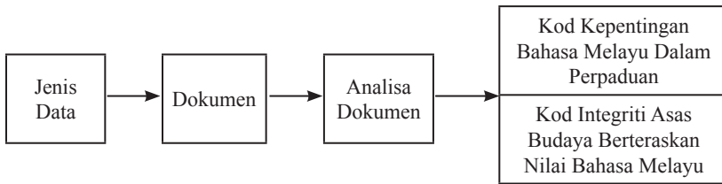
Rajah 1 Carta Alir Penganalisisan Data
